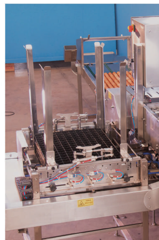
Dispensador de bandejas plásticas (denester) lateral
